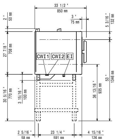
Zij aanzicht
